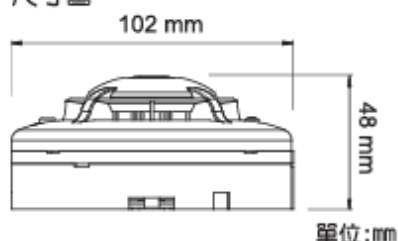
尺寸圖
