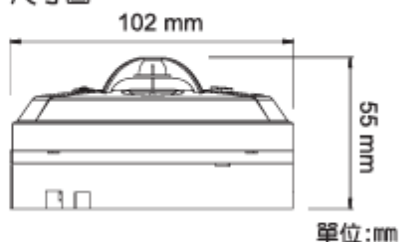
尺寸圖
