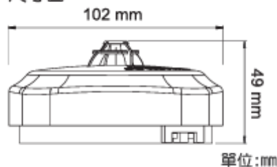
尺寸圖
